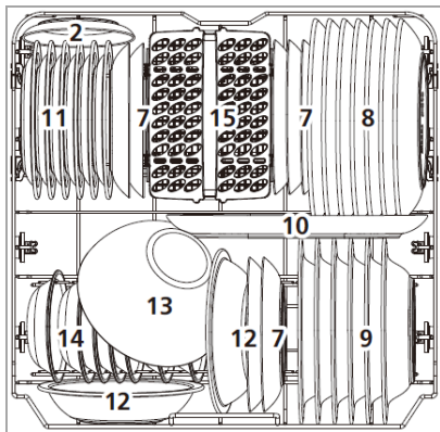
Beladung unterer Korb gemäß EN60436
