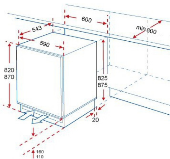
Einbauskeizze
